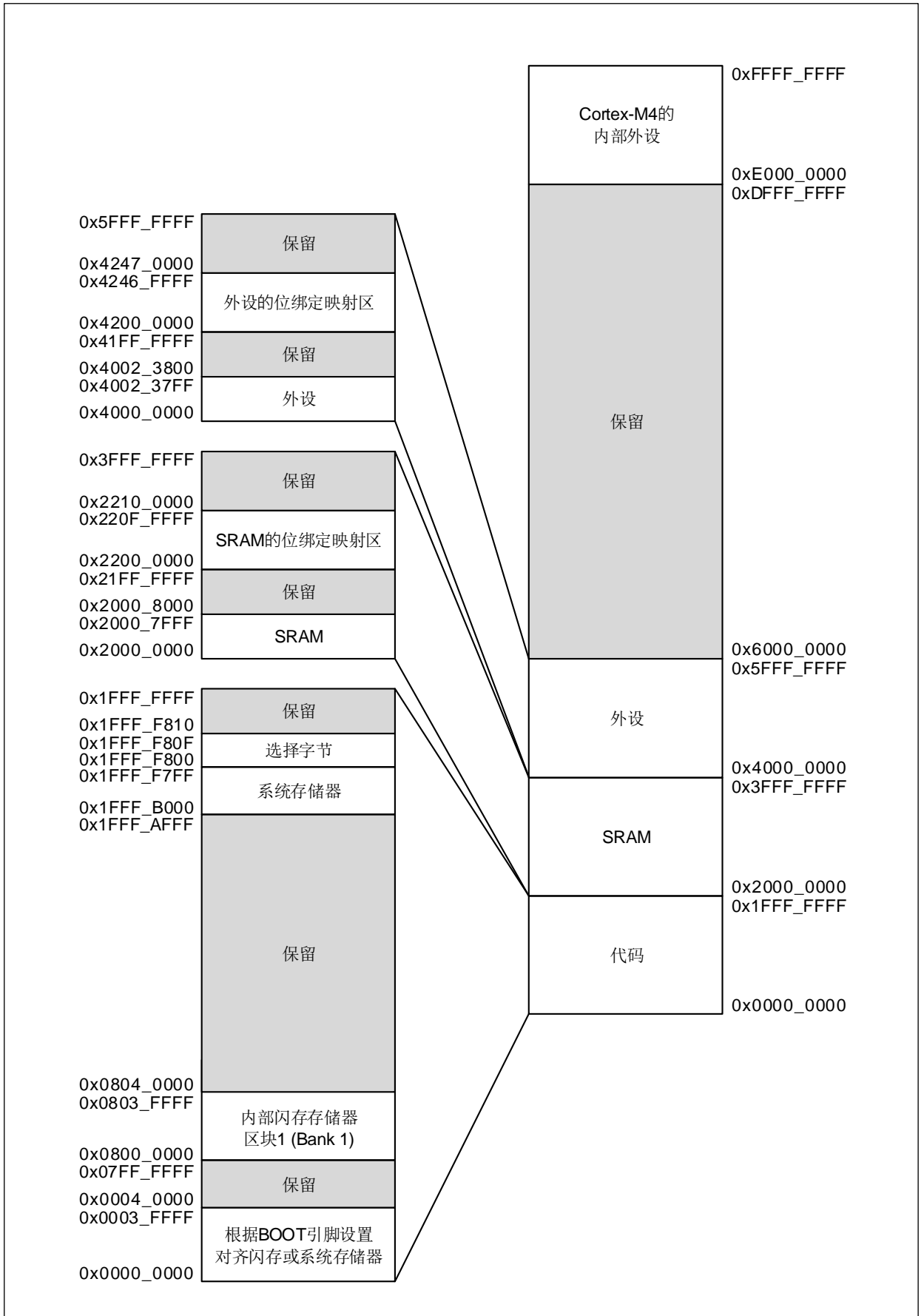
图 7. 存储器图
