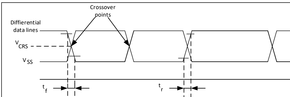
图 25. OTGFS 时序：数据信号上升和下降时间定义
