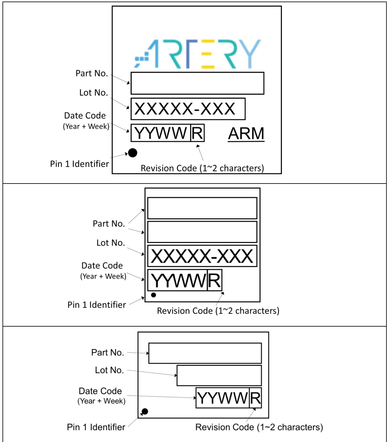
图 35. 丝印示意图
