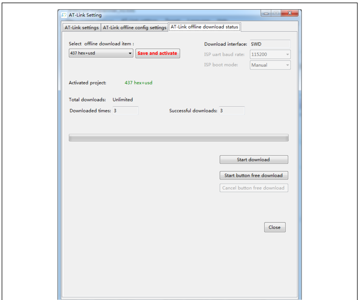
图 23. 离线下载界面
