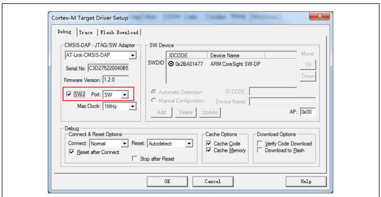
图 8. Keil 的 Debug settings 配置
