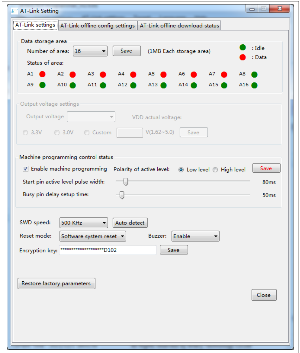
图 17. 参数设置界面
