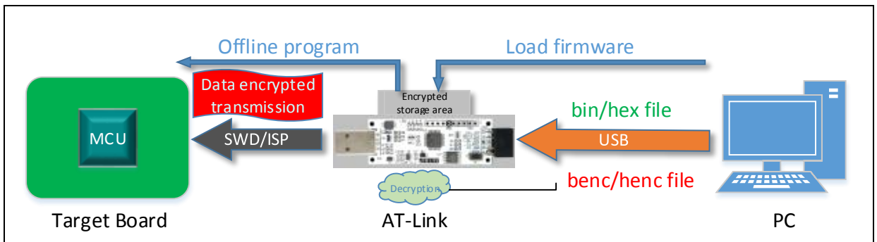
图 21. 离线编程流程图
