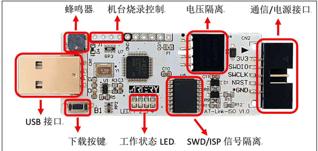
图 4. AT-Link-ISO 硬件外观接口
