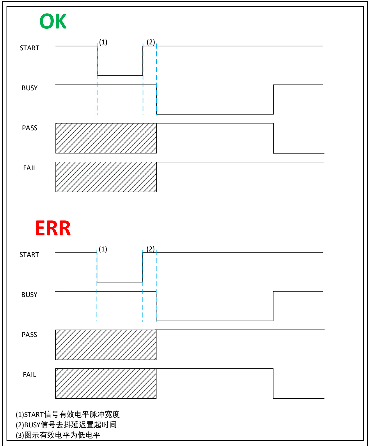
图 26. 机台烧录控制典型时序图
