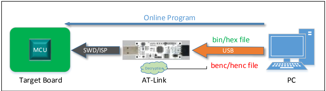
图 18. 在线编程流程图
