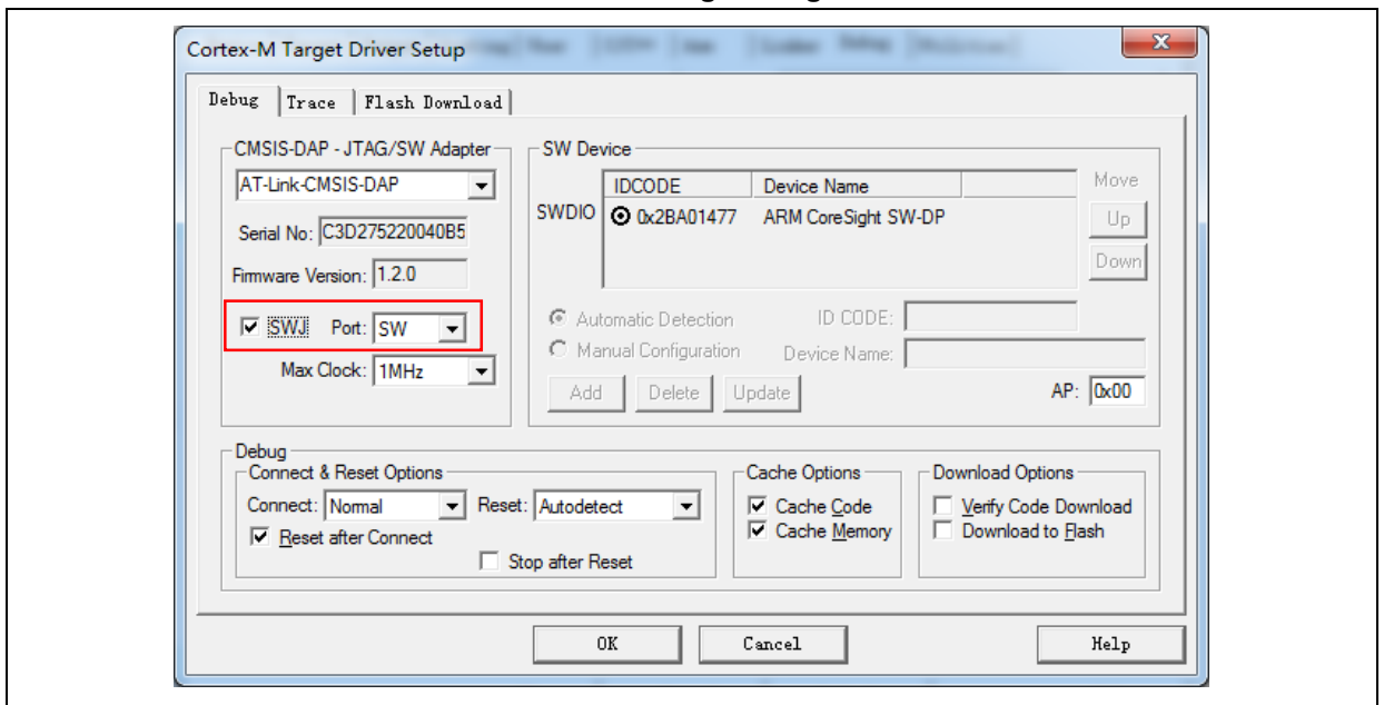
图 8. Keil 的 Debug settings 配置
