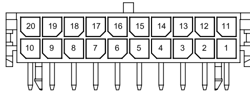
20-CKT.
