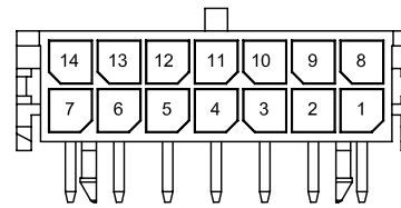
14-CKT.
