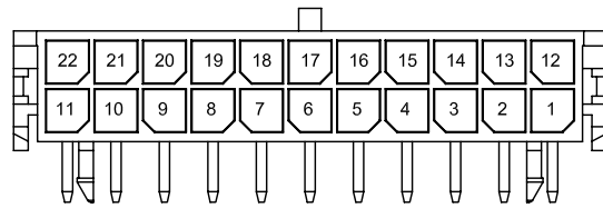
22-CKT.
