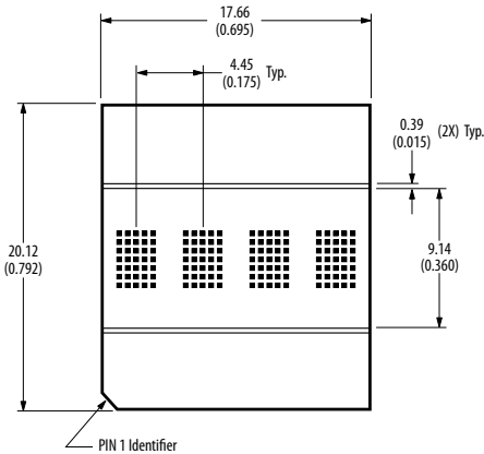
HDLx-1414
