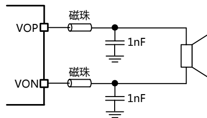
图 7 磁珠与电容
