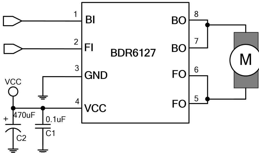
图 4. 应用原理图
