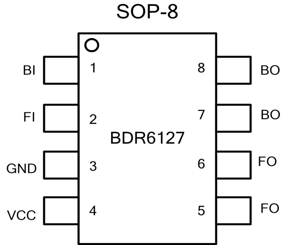
图 2. 顶视图
