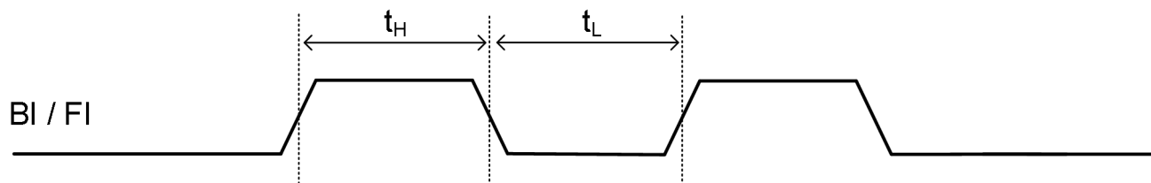
图 5. 输出时序图
