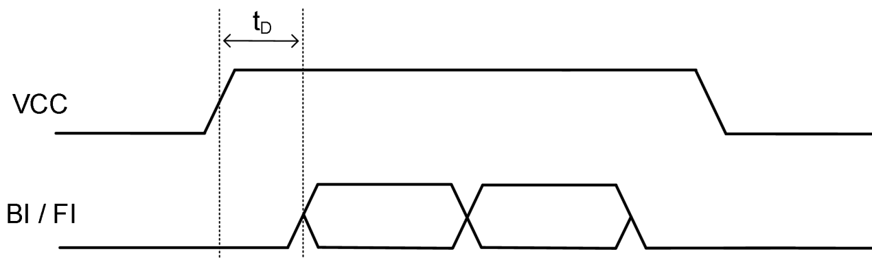
图 6. 上电时序图
