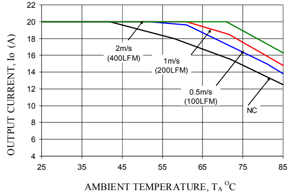
Vo=1.2V
