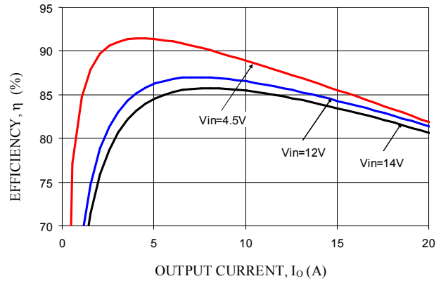
V_o = 1.2V
