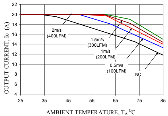
Vo=5.0V
