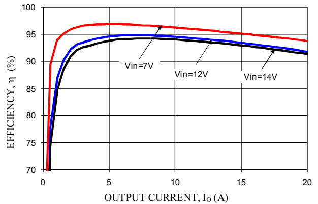
V_o = 5.0V
