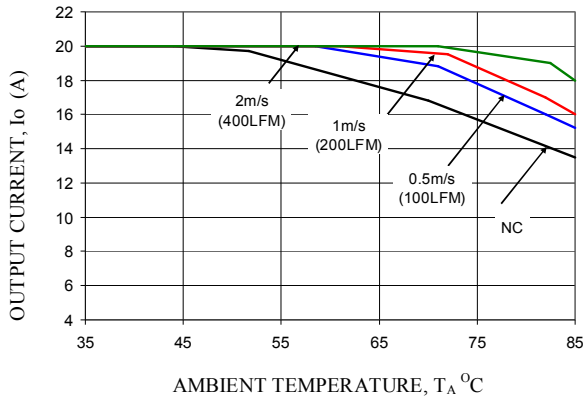
Vo=0.69V
