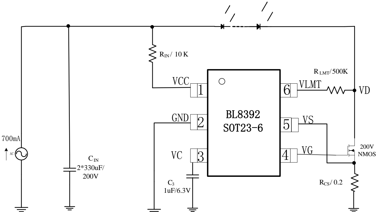
图 1: 典型应用图
