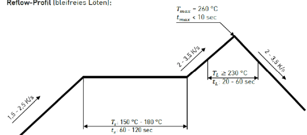
Reflow-Profil (bleifreies Löten):
