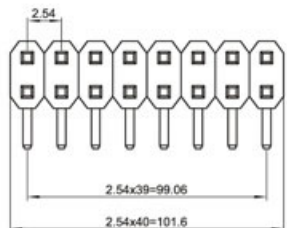
Terminal(Du Pont2.54)
