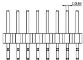
Du Pont2.54-2xnAW
