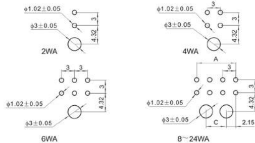
针座 WAFER (43045)
