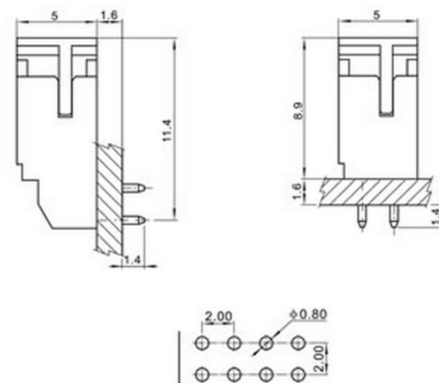
P.C.B. LAYOUT
