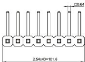
Du Pont 2.54-nAW
