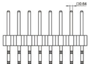
Du Pont 2.54-2xnAW
