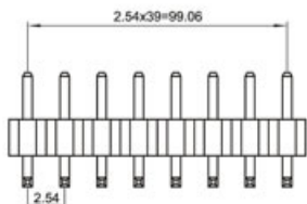
Du Pont 2.54-PT
