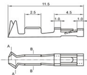
Du Pont 2.54-PT
