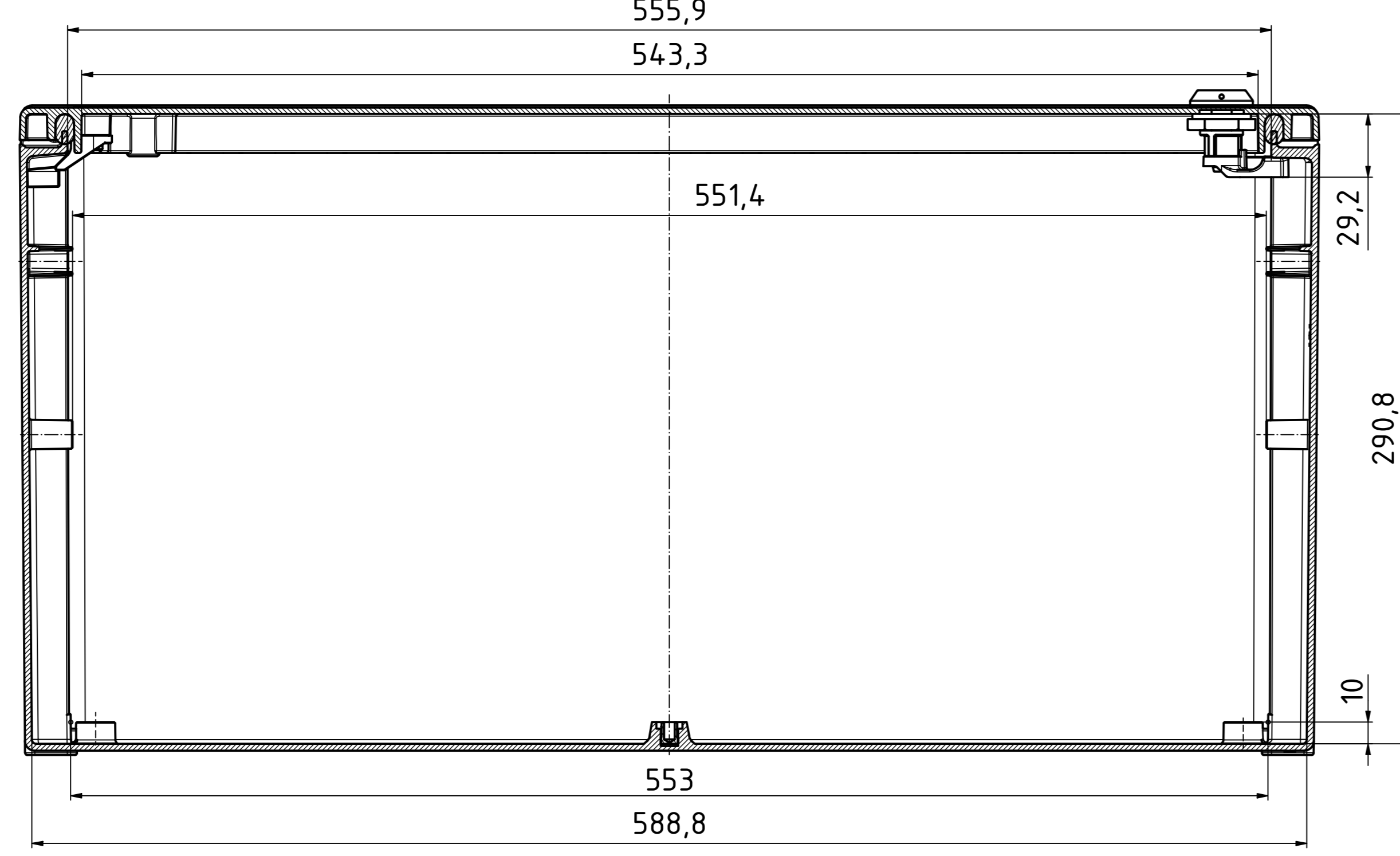
A-A ( 1 : 2 )
