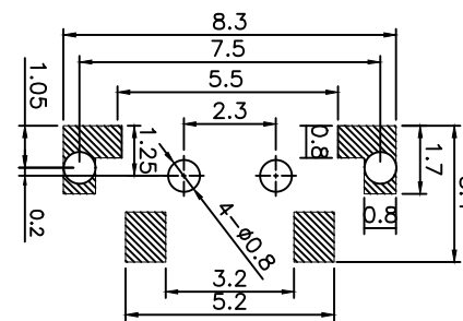
PCB. 焊接图
