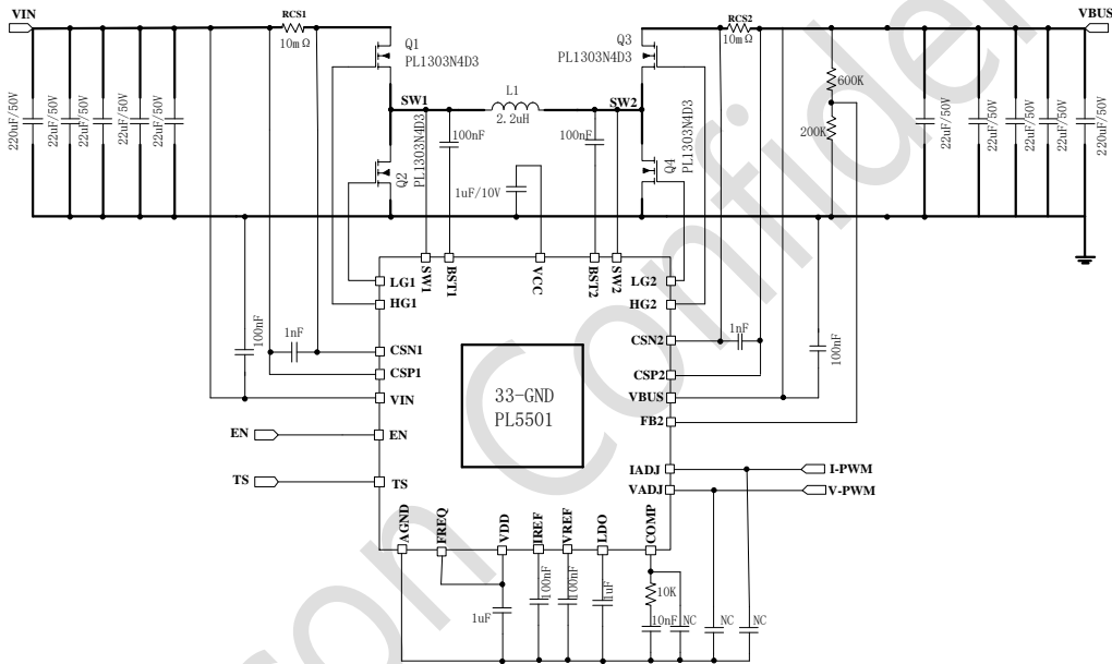
Fig. 31 Schematic
