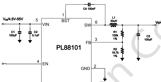
Fig. 1 Schematic
