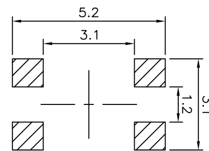
PCB. 焊接图
