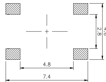
PCB. 焊接图
