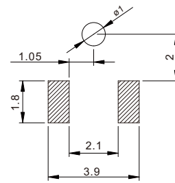
安装图 instructions
