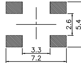
PCB. 焊接图
