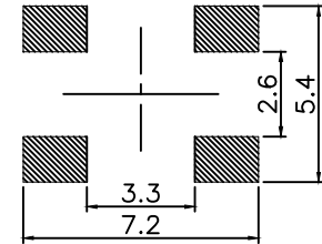
PCB. 焊接图
