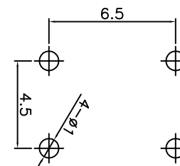
PCB. 焊接图
