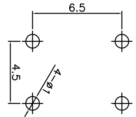
PCB. 焊接图
