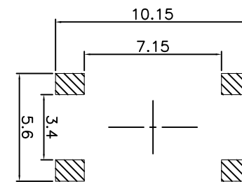
PCB. 焊接图
