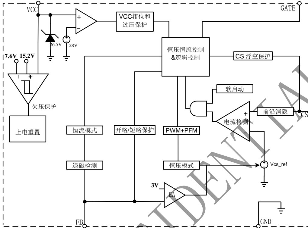
图 3 BP2519 内部框图
