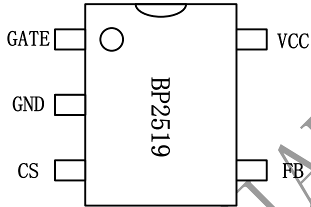
图 2 管脚封装图
