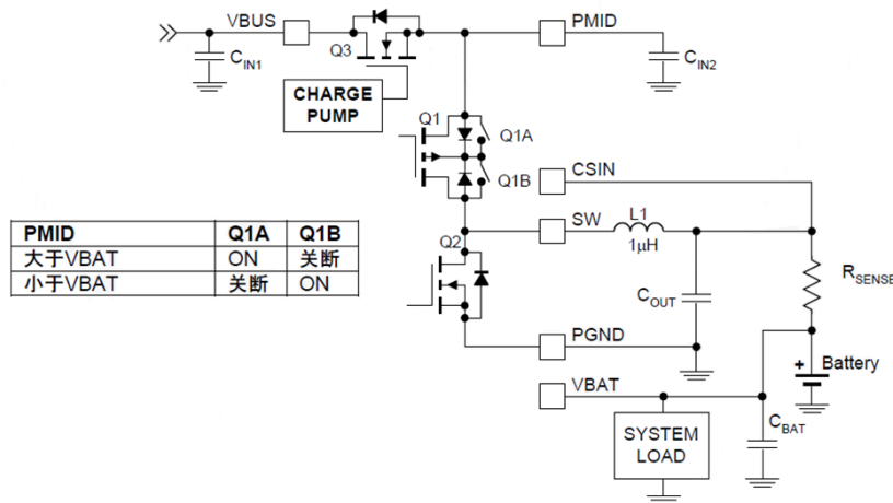
图 4 功率级
