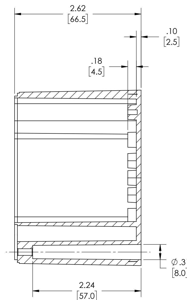
SECTION A-A
