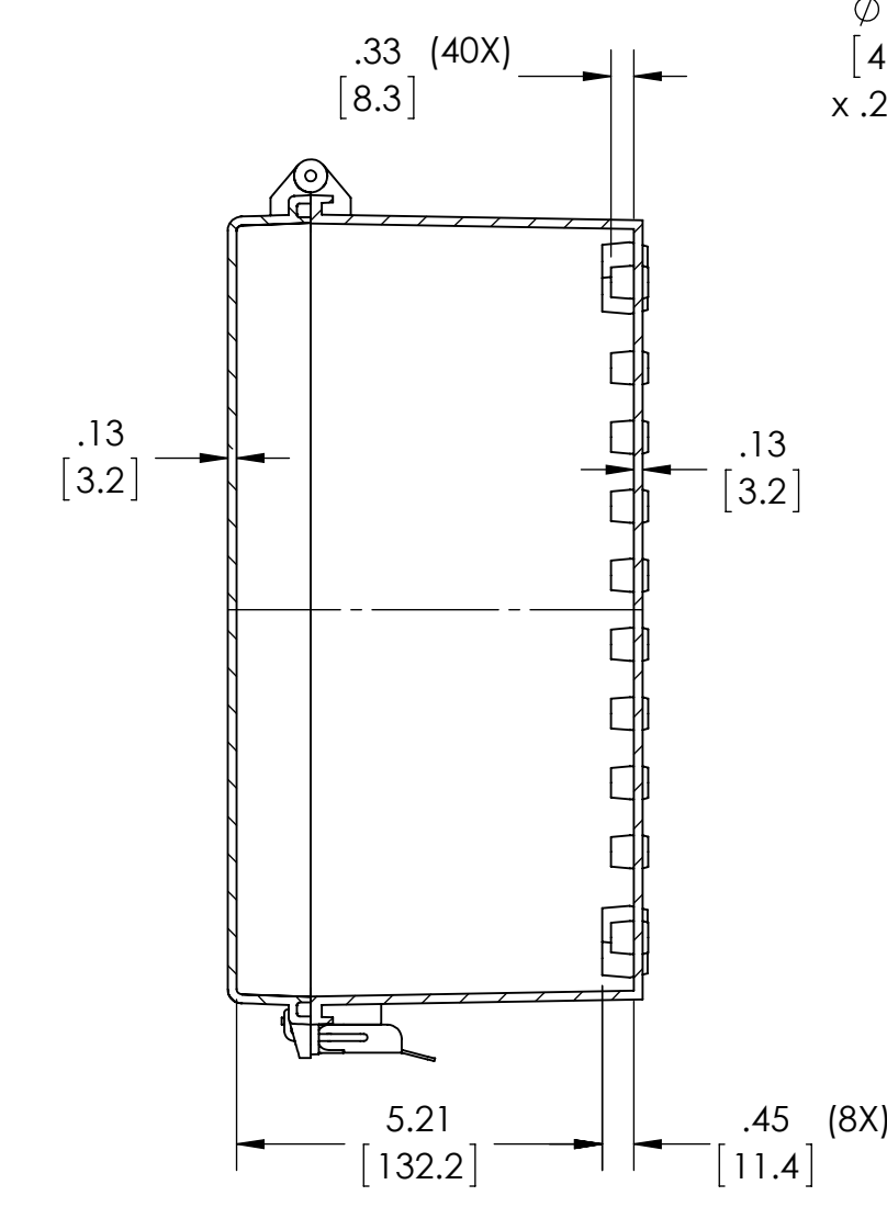
SECTION A-A SCALE 1 : 3
