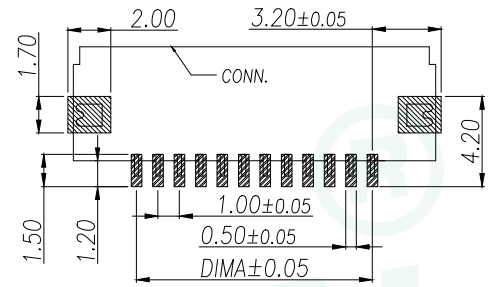
通用线路板(PCB LAYOUT)
