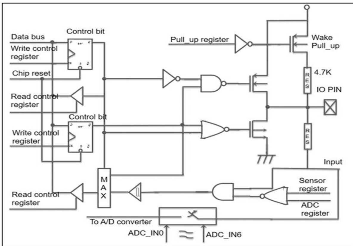
ADC 结构图
