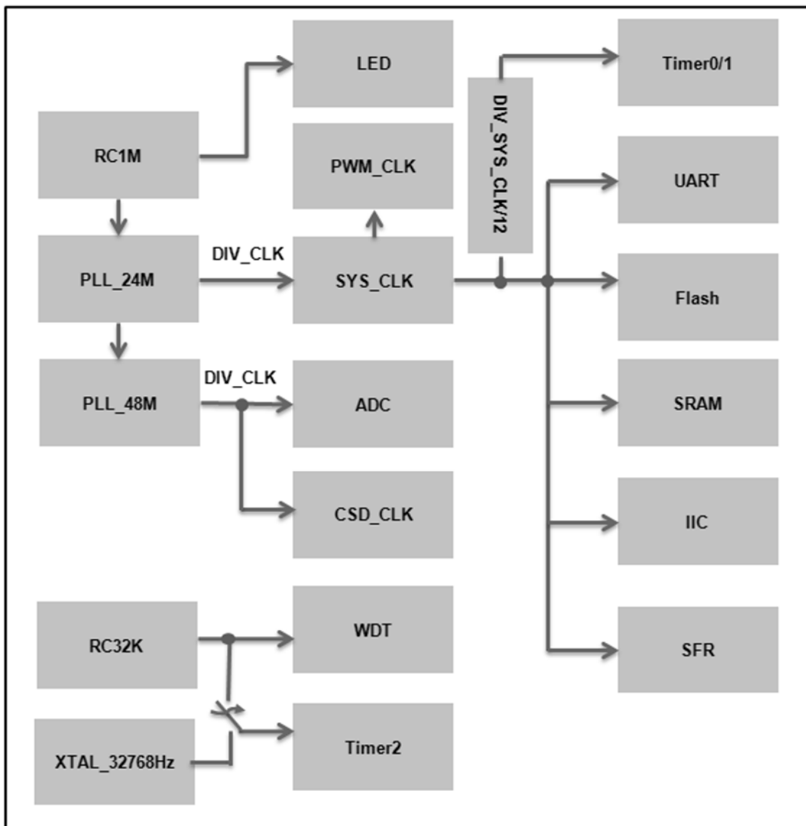
时钟分布图
