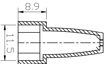
剖视图
