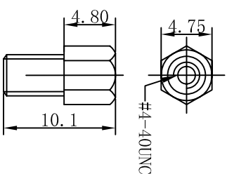
螺丝示意图
