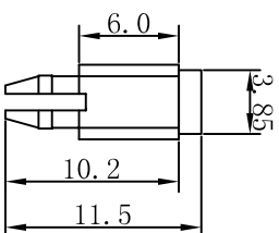
铆钉示意图
