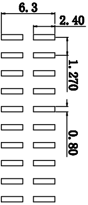
P. C. B. LAYOUT
