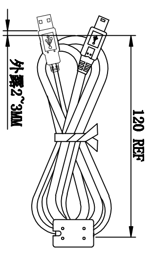
绕线图示
