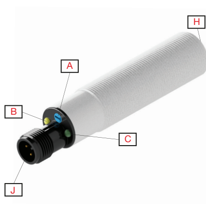
Fig. 2 CA18 Plug
