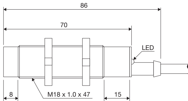
Fig. 7 Cable CA18EAN...A2IO
