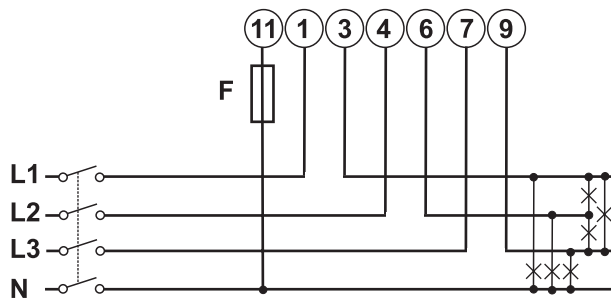
Fig. 30 AV2, AV9
