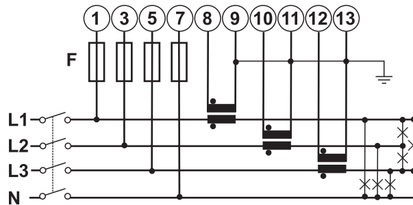
Fig. 31 AV5, AV6
