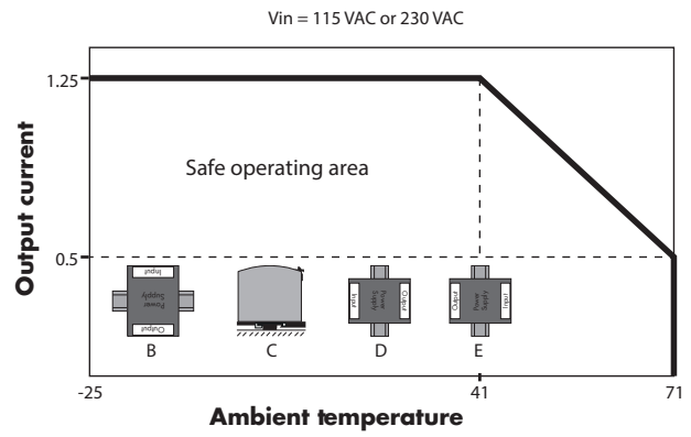
SPDM 30W / 24VDC
