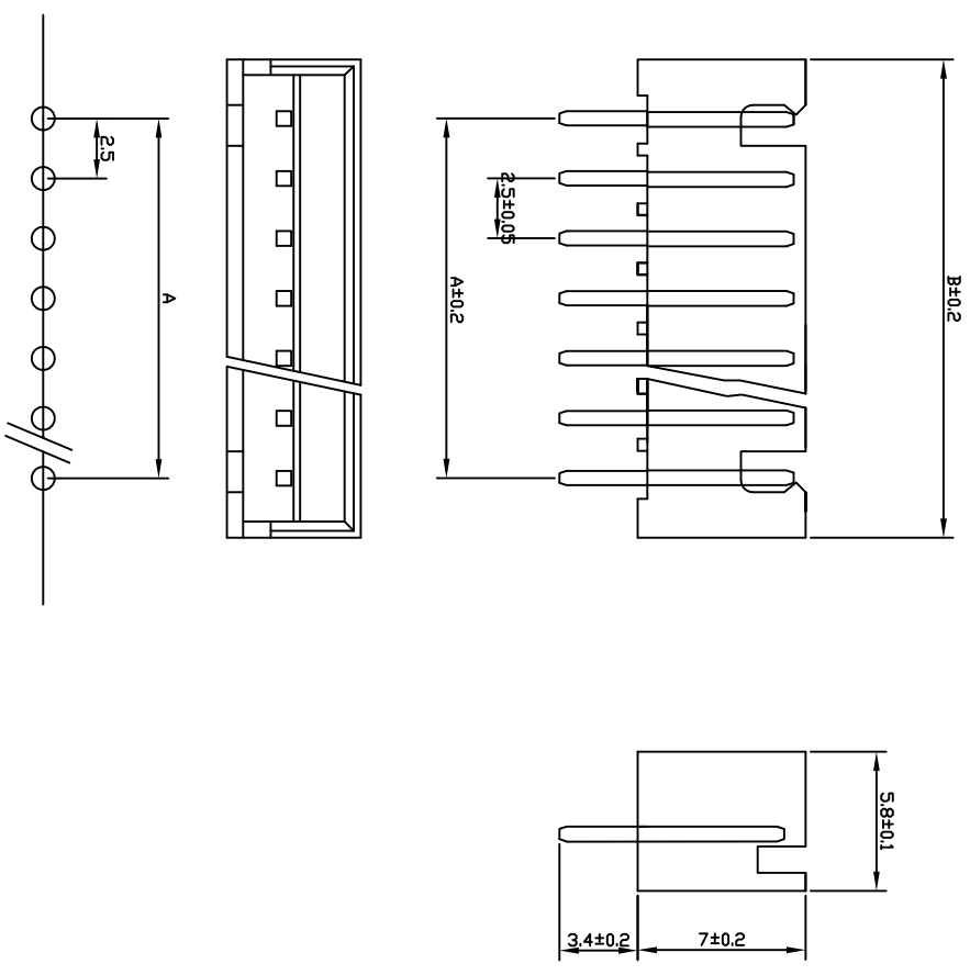
PCB寸法
