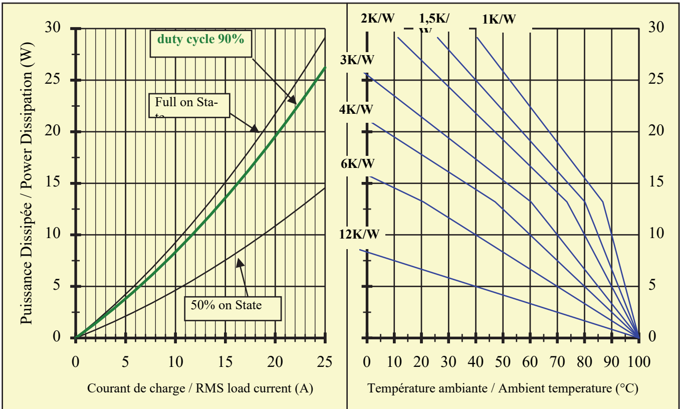
Courbe de puissance dissipée en fonction du courant commuté et du cycle de marche, de la résistance thermique du dissipateur et de la température ambiante. Power Dissipation curve in compliance with nominal load current, ON/OFF duty cycle, thermal resistance of the heatsink and ambient temperature.
