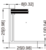
Section A-A
