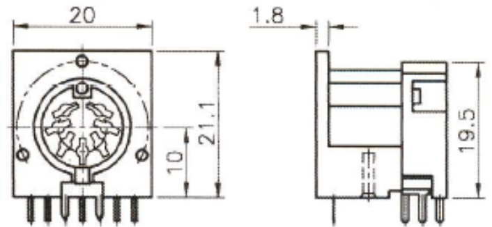
DS-027 / DS-028
