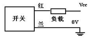
直流二线接线方式
