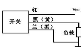
PNP 接线方式
