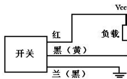
NPN 接线方式
