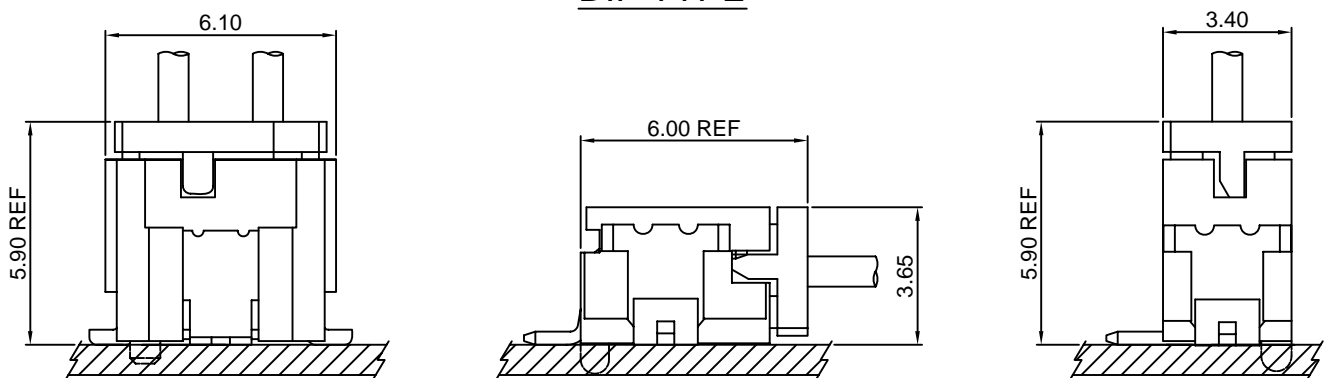
SMT TYPE
