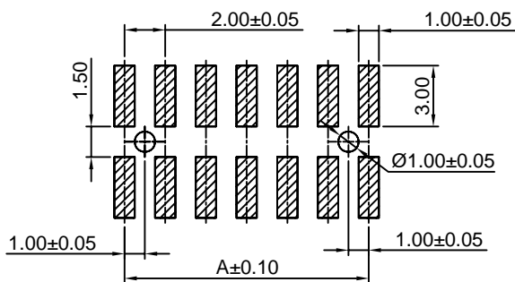
P.C.B LAYOUT
