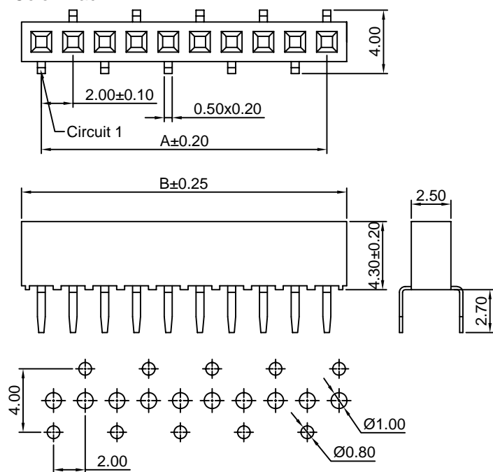
P.C.B LAYOUT
