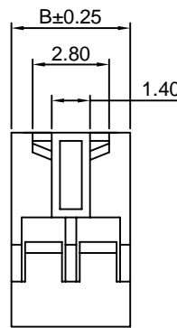
2x2P
