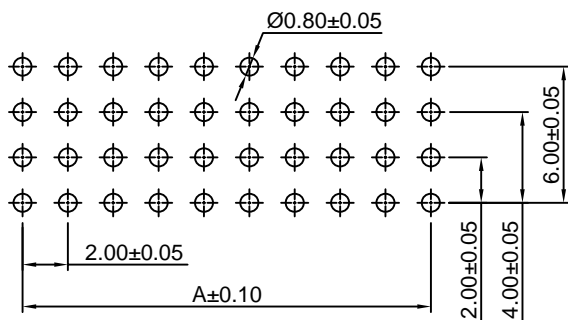
P.C.B LAYOUT
