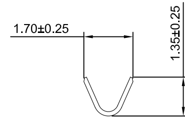
SEC:B-B
